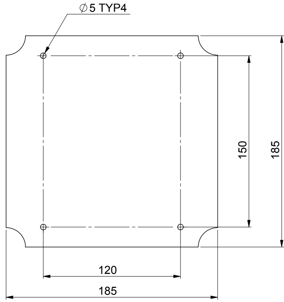
SCALE 1 : 2
